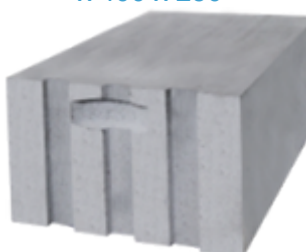
Блок газобетонный с пазом, гребнем и захватом для рук 625 x 400 x 250
